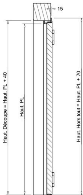
Coupe B-B
