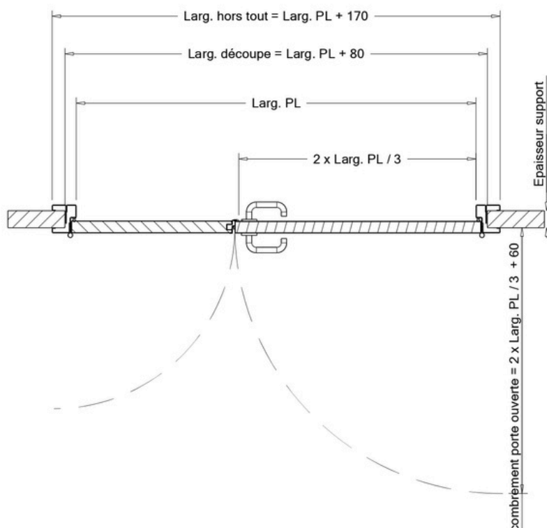
Coupe A-A
