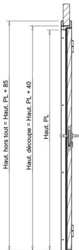
Coupe B-B
