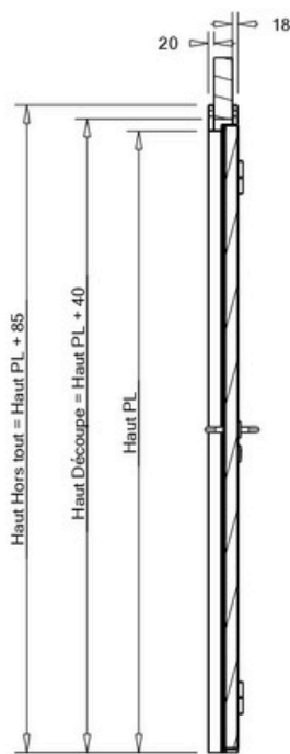
Coupe B-B
