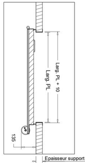
Coupe A-A
