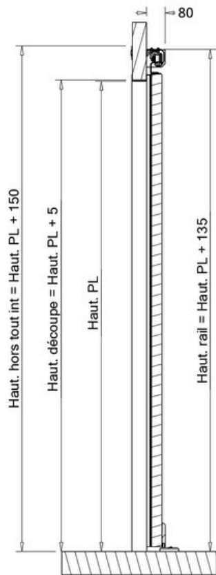
Coupe C-C
