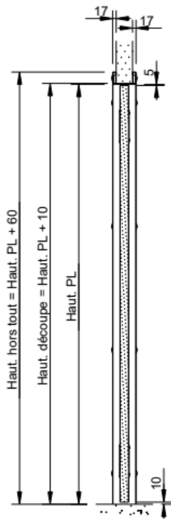
Coupe B-B
