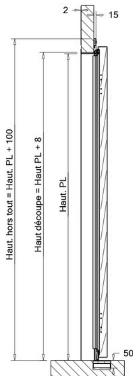
Coupe B-B
