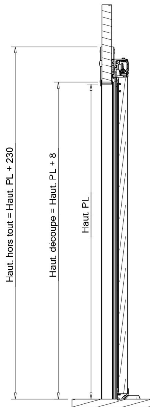
Coupe C-C
