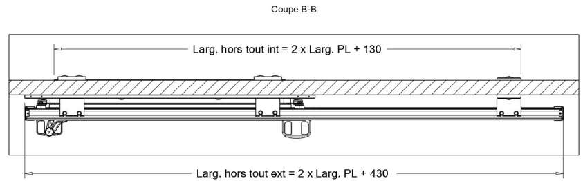
Coupe B-B
